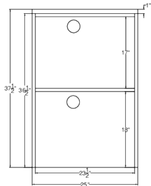
Elev
